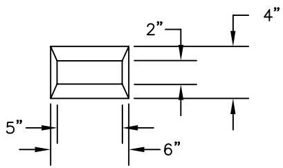
TYP. HOLE DET.
